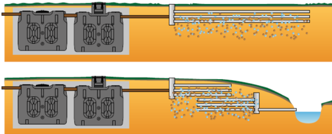
Ejemplo de instalación de arquetas de repartición.
